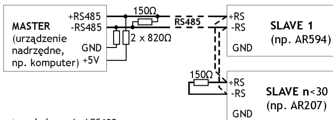
Rys.17. Schemat poglądowy sieci RS485
