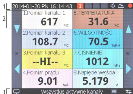
Rys.11.2. Wygląd ekranu grupy pomiarów w trybie TYLKO TEKST (możliwość prezentacji maksymalnie 8 kanałów)
